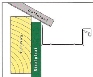
Aluminium dakgoot bevestigd aan de geprofileerde staalplaat.
