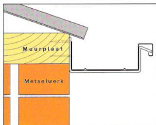
Gemonteerd aan de muurplaat met metselwerk.
