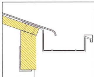
Aluminium dakgoot bevestigd aan het dakbeschoot.
